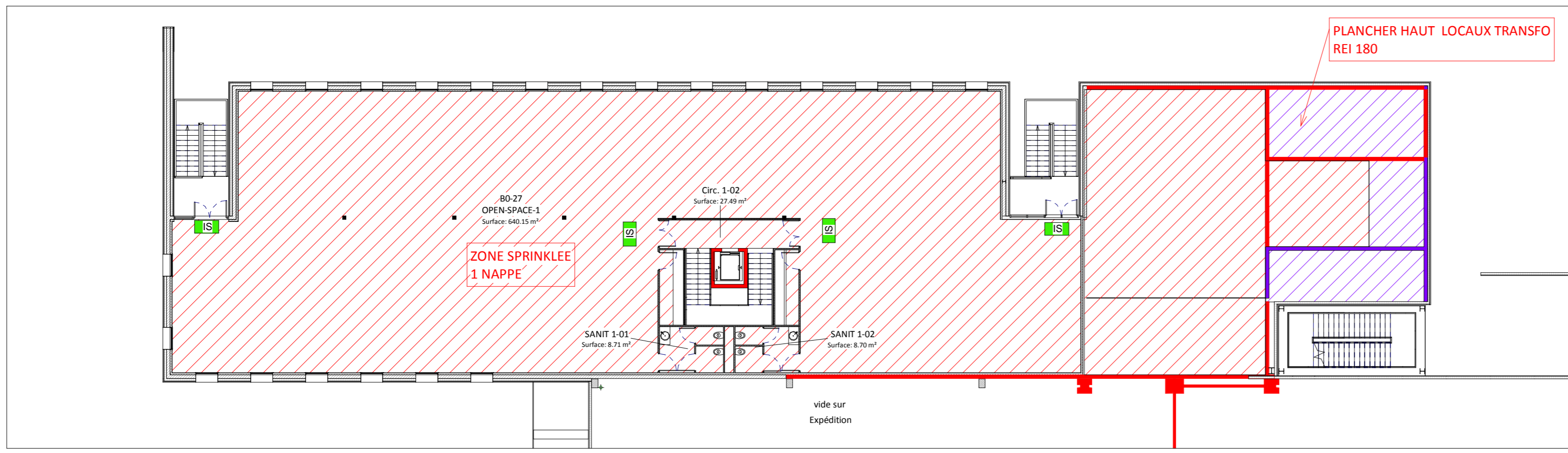
SI NIVEAU +3.60 Ech : 1 : 200
