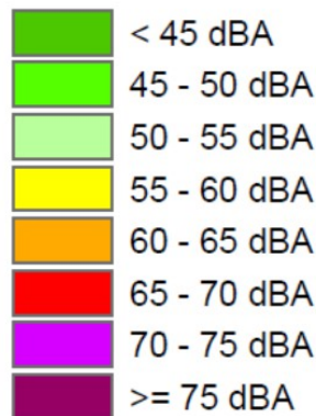
Illustration 3 : Classe de bruit et code couleur issus de la norme NF S 31-130
